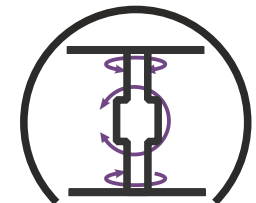
Подложкодержатель для пластин \varnothing 150 мм
